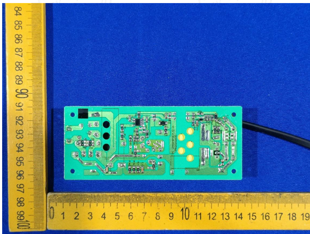
照片 15 内部电源
