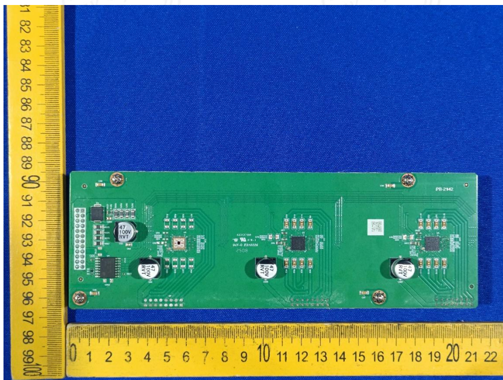
照片 13 内部 PCB
