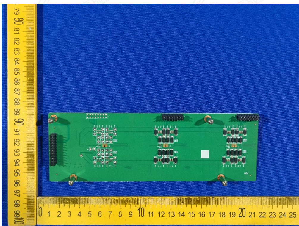
照片 12 内部 PCB
