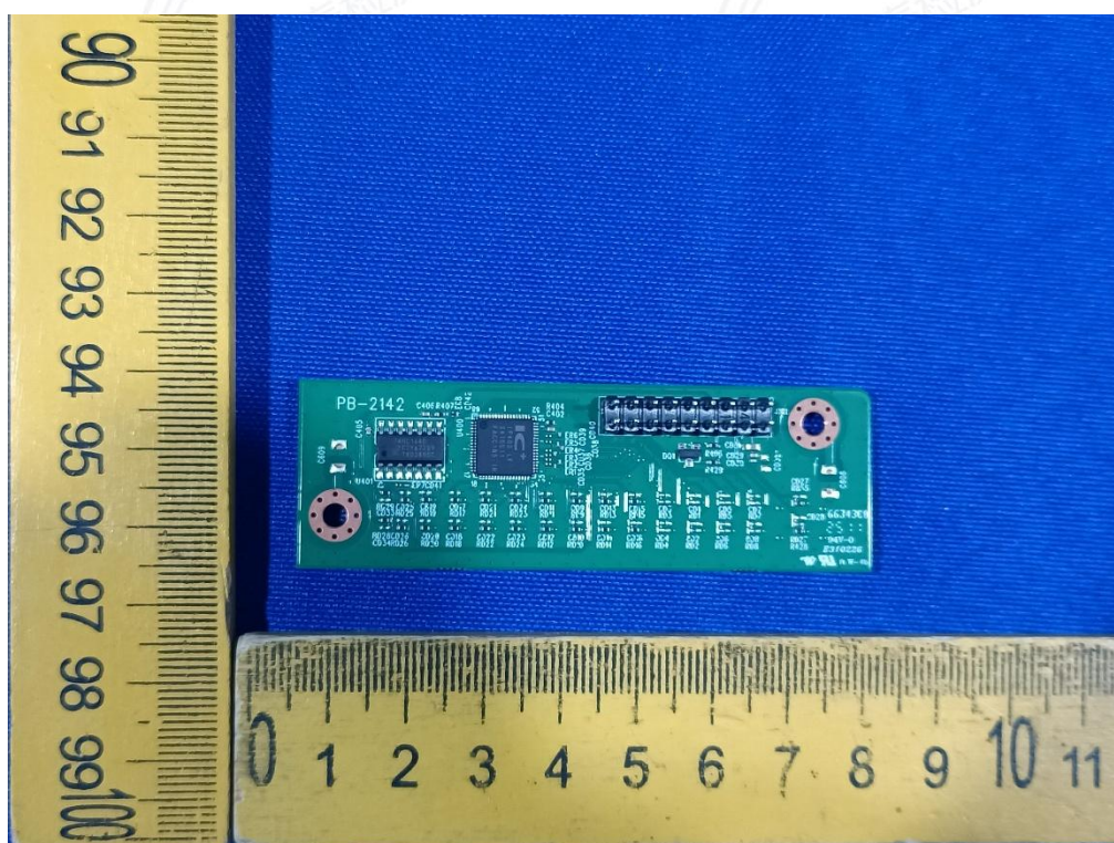
照片 16 内部 PCB
