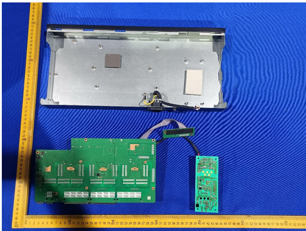
照片 7 内部视图
