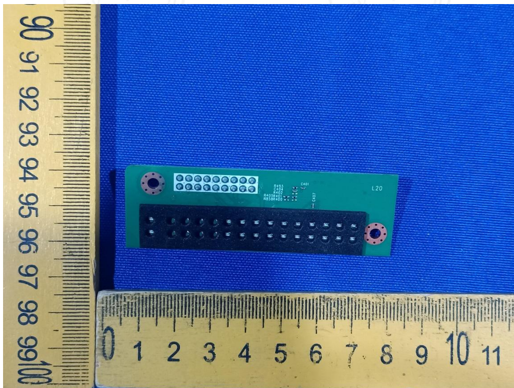
照片 17 内部 PCB
